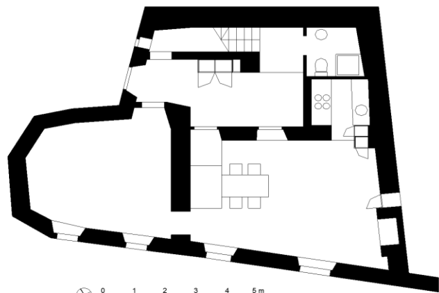
Pian terreno 0 1 2 3 4 5 m
